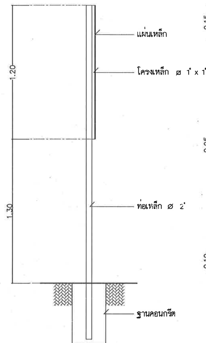
รูปด้านข้าง มาตรฐาน 1 : 20
