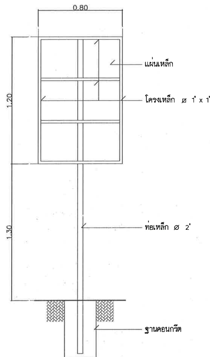
รูปด้านหลัง มาตรฐาน 1 : 20
