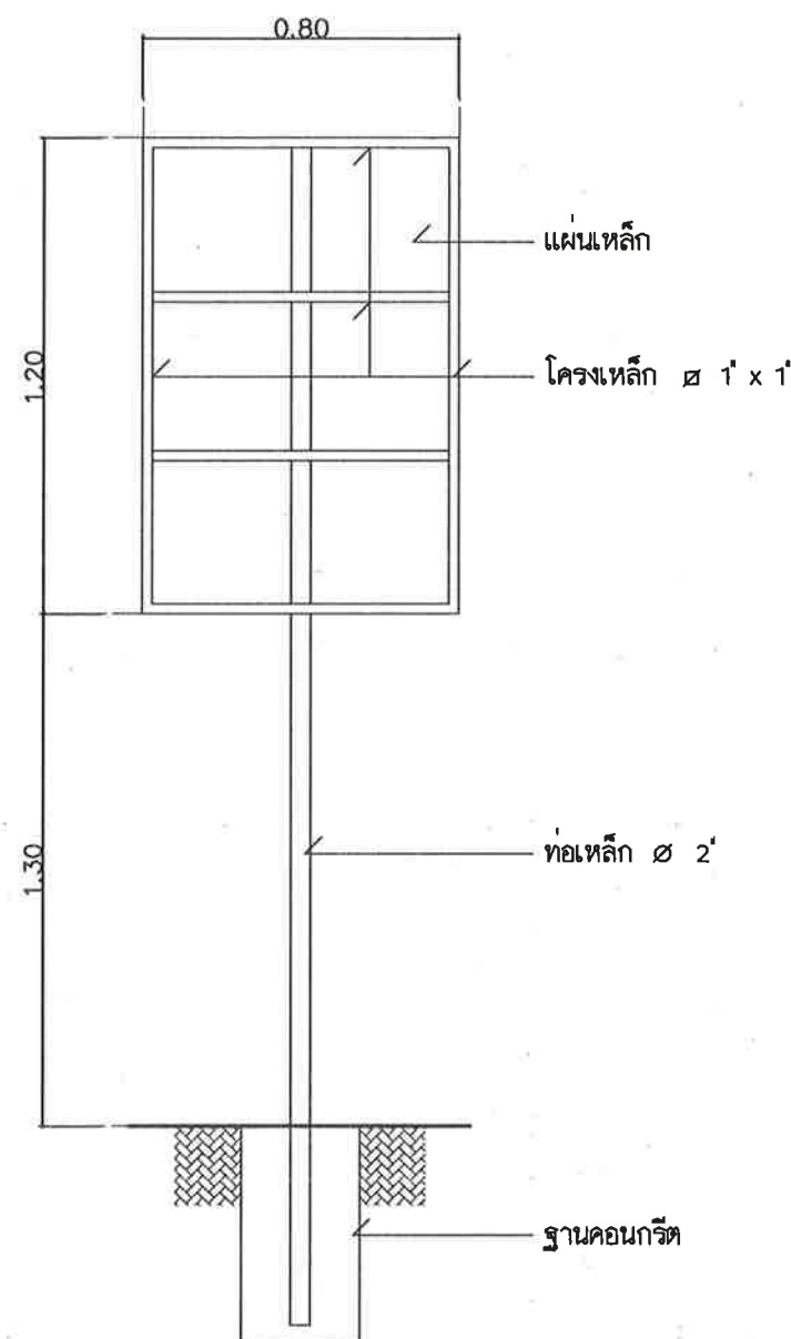
ด้านหลัง มาตรฐาน 1 : 20
