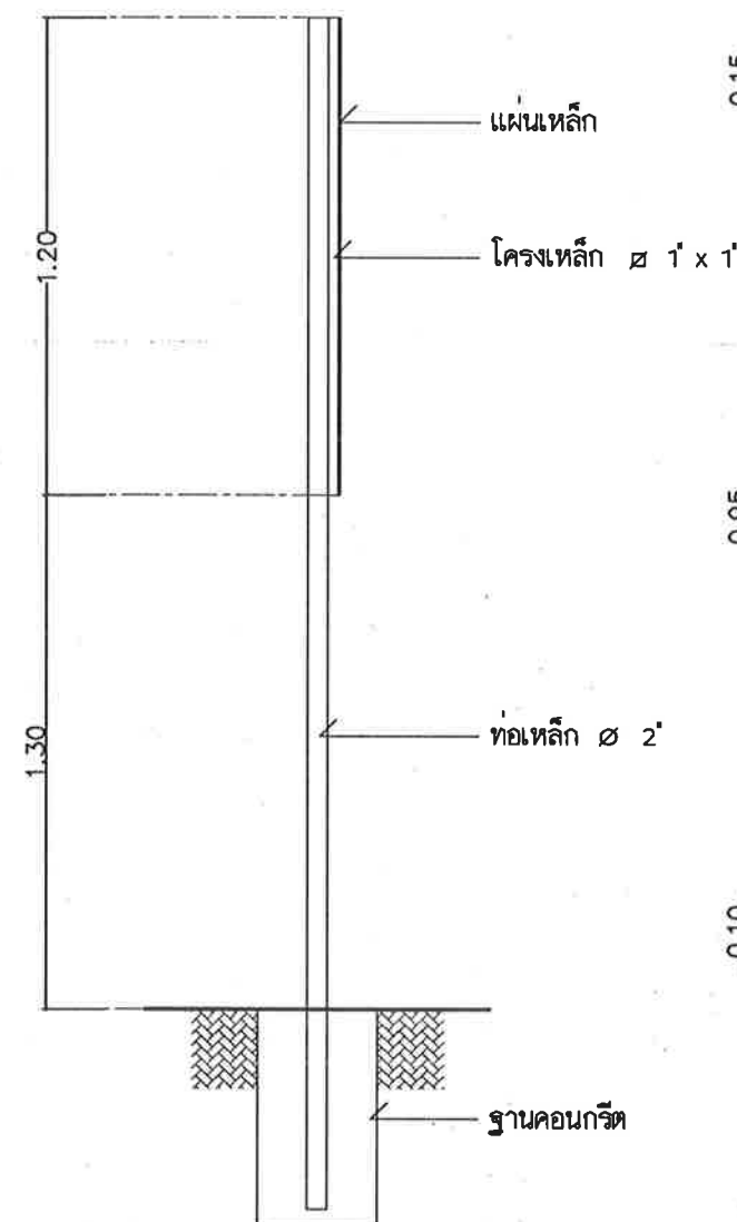
ด้านข้าง มาตรฐาน 1 : 20
