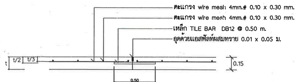
แบบขยาย ค LONGITUDINAL JOINT 1 : 25
