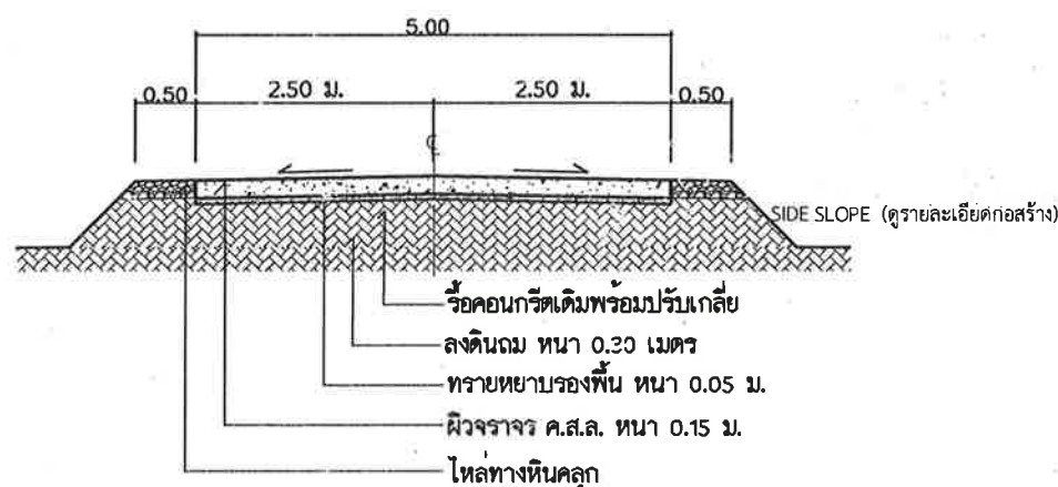
รูปตัด 1 : 75
