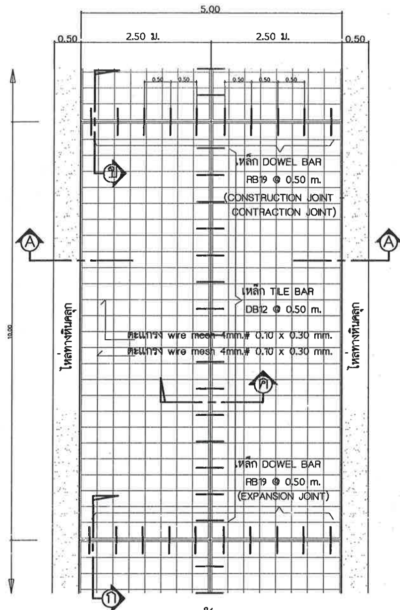
แปลนพื้นถนน 1 : 75
